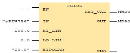
Рисунок 1- Ввод данных датчика температуры
