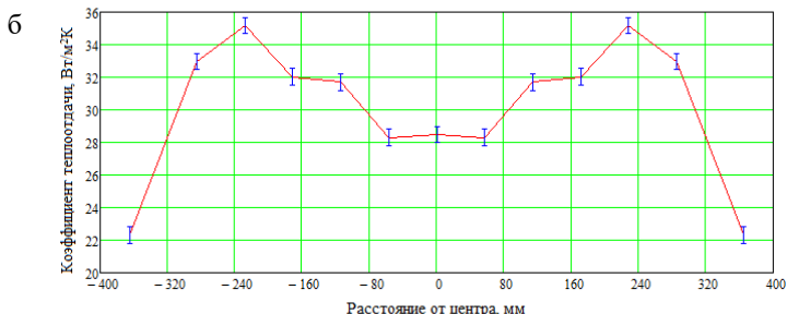
Рис. 1. Распределение коэффициента теплоотдачи и оценка погрешности измерения: а – по высоте факела на вертикальной оси; б – по ширине факела на горизонтальной оси
