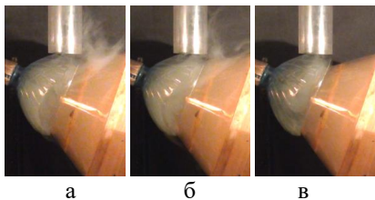
Рисунок 3 – Характерные картины распределения потоков дыма при имитации газоотсоса центробежным вентилятором
