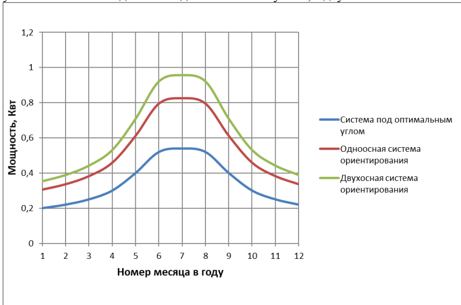
Рисунок 1 - График максимальной мощности на 1 м 2 в зависимости от месяца
