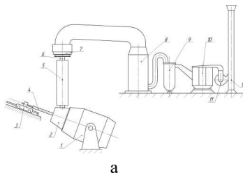
а б Рисунок 2 – Структурная схема модернизированной системы газоотсоса кислородного конвертера с вращающимся корпусом (а) и общий вид модельного комплекса
