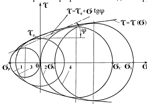
Рис. 1 – Графическая интерпретация теории Кулона-Мора в детерминированной постановке:
