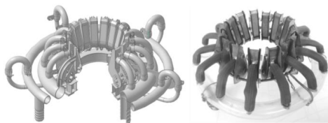
Рисунок 1 – 3D и действующая модель предложенного вентилятора
