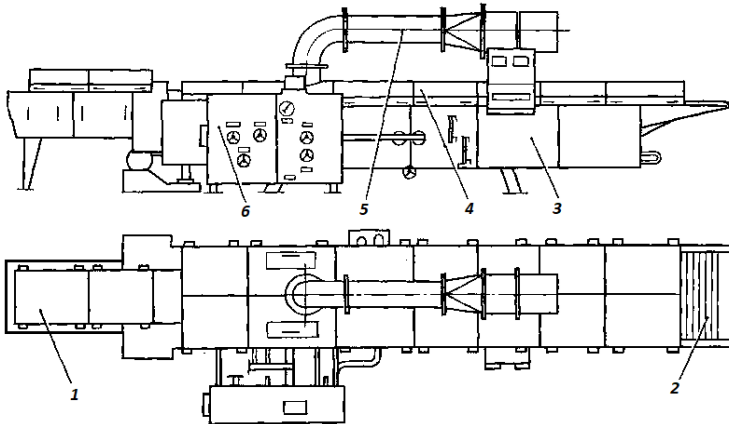
Рисунок 1 - Обжарочная печь конструкции ЦПКТБ «Азчеррыбы»
