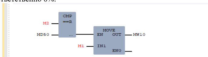
Рисунок 2 - Сравнение реальных значений с табличными
